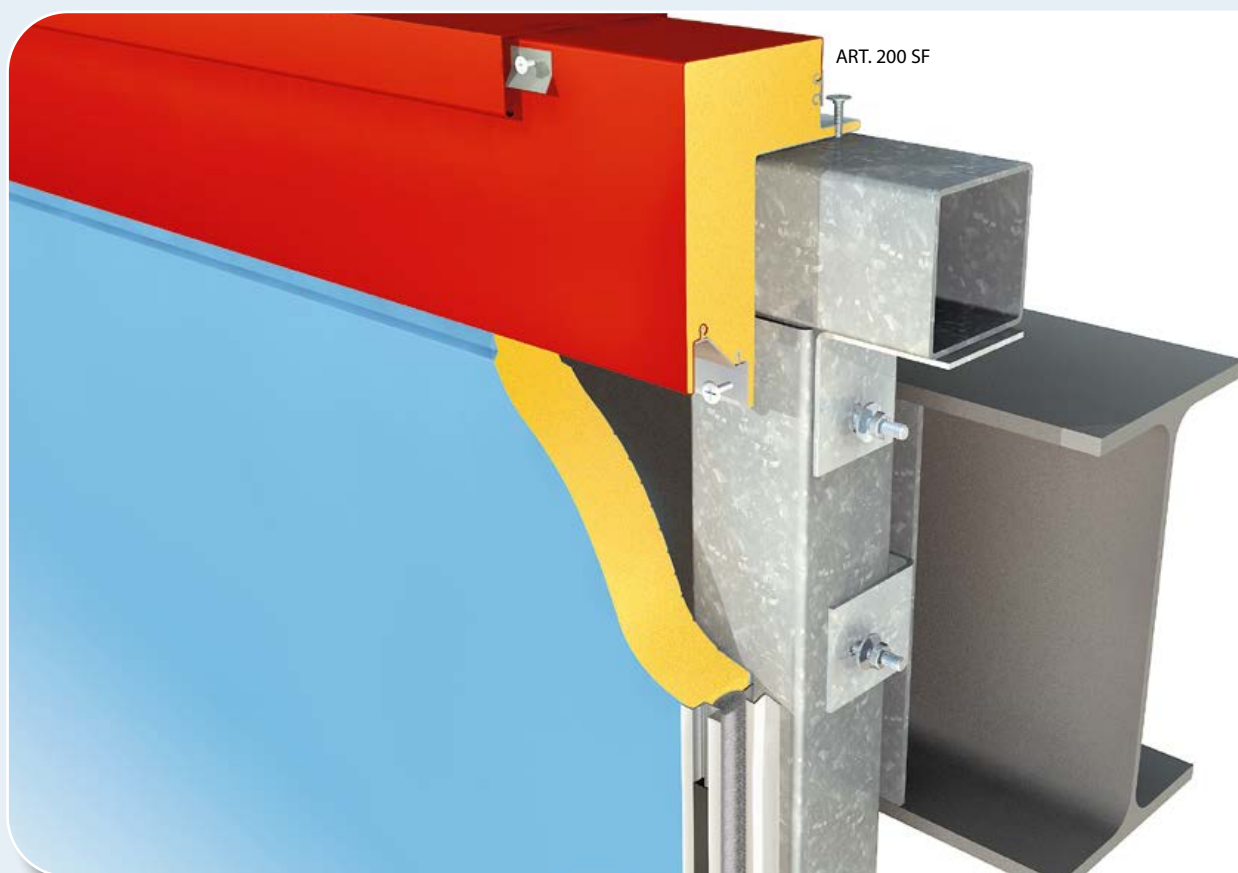
CORONAMENTO SUPERIORE ANGOLO 90° FOAMED 90° UPPER CONNECTION
