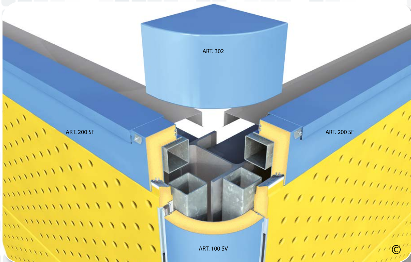
ANGOLI CURVI VERTICALI / ANGOLI RETTI ORIZZONTALI CORONAMENTO SUPERIORE ROUNDED VERTICAL CORNERS / HORIZONTAL 90° CORNERS, UPPER CONNECTIONS
